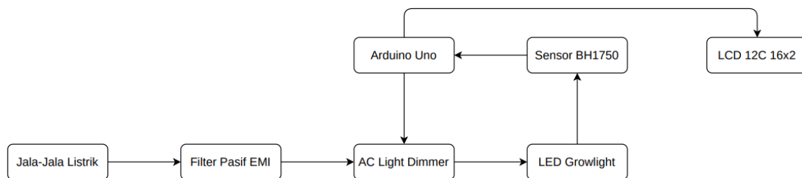
Gambar 1. Diagram Blok Sistem
